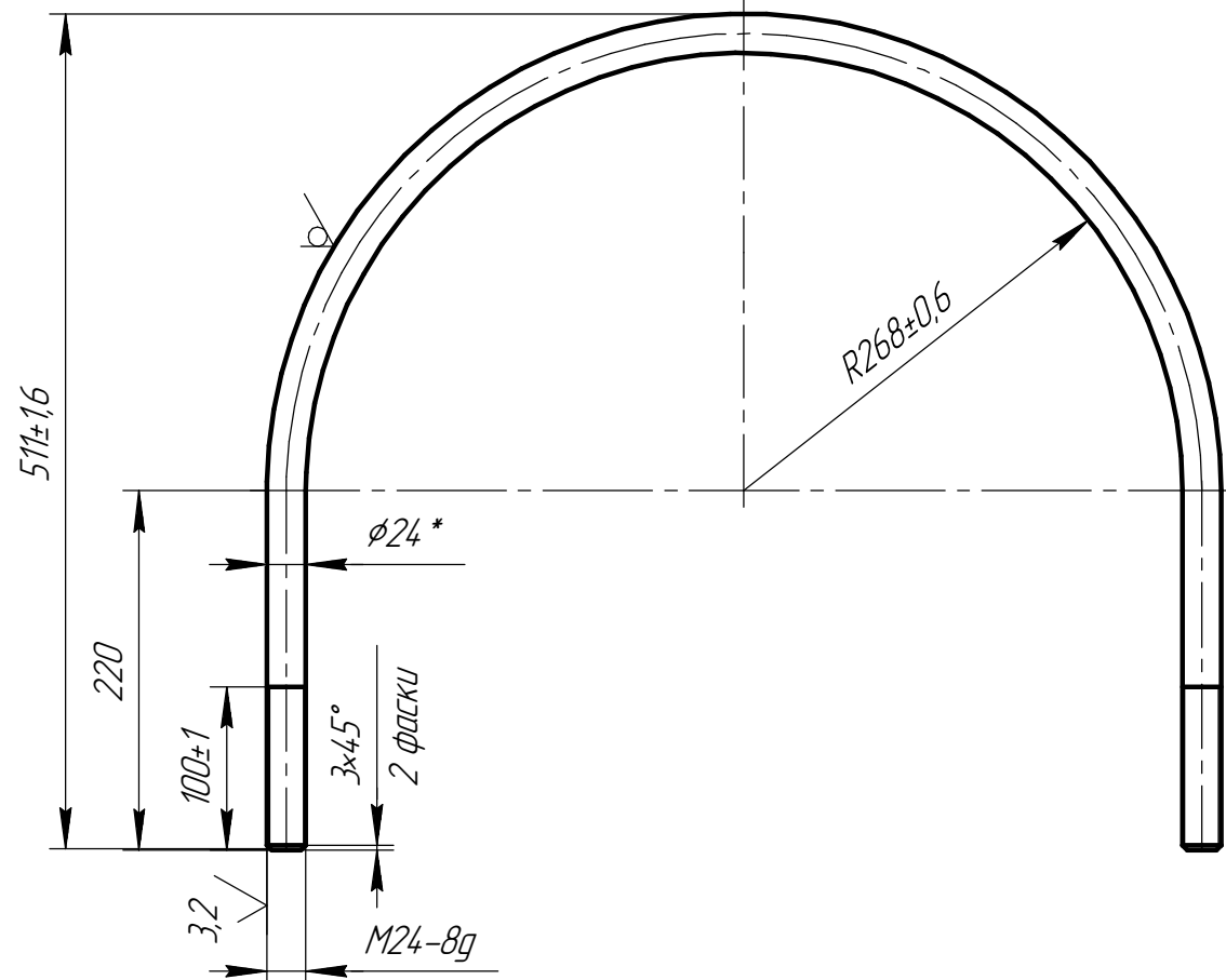
Дет. поз. 5
