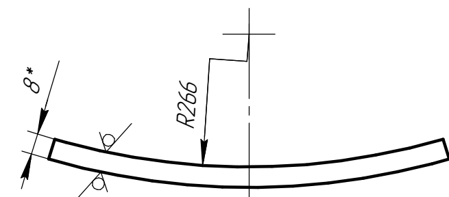
Дет. поз. 6 (1:2)
